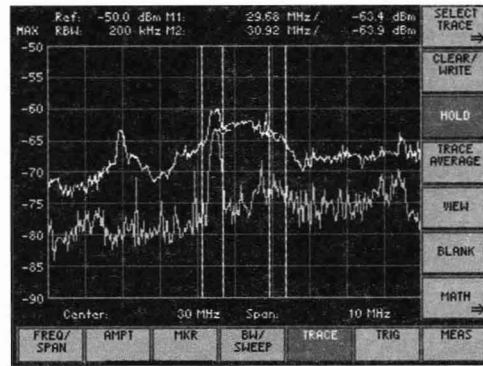
Рис. 6. Поле ЭМИ конденсаторной С-антенны
