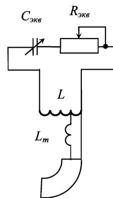
Рис. 4. Схема подключения эквивалента конденсаторной С-антенны при измерении сопротивления излучения
